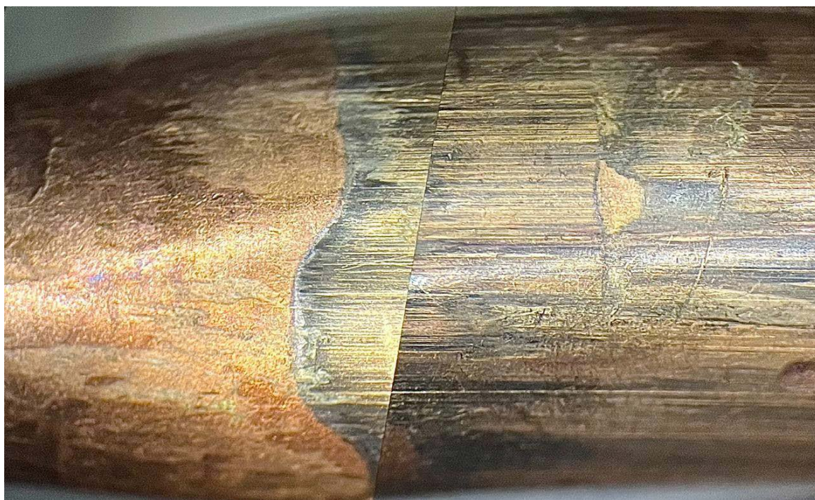
Фото. 4. Совмещение следов полей и нарезав канала ствола на оболочечных пулях FMJ, выстреленных в охотничьем карабине АК–366 Ланкастер кал. .366 ТКМ Fig. 4. Combining traces of rifling lands and rifling of the barrel bore on FMJ shell bullets fired in the AK–366 Lancaster cal hunting carbine. .366 TCM
