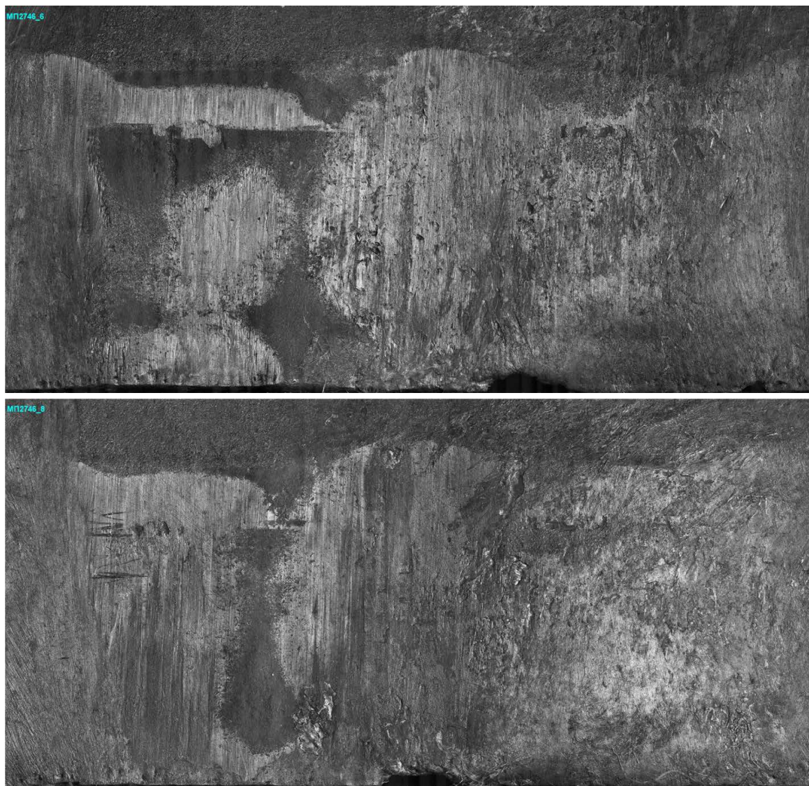
Фото 5. Следы сверловки «Ланкастер» на ведущей части выстреленных пуль (охотничий карабин АК–366 Ланкастер кал. .366 ТКМ, пуля «ЭКО»)
